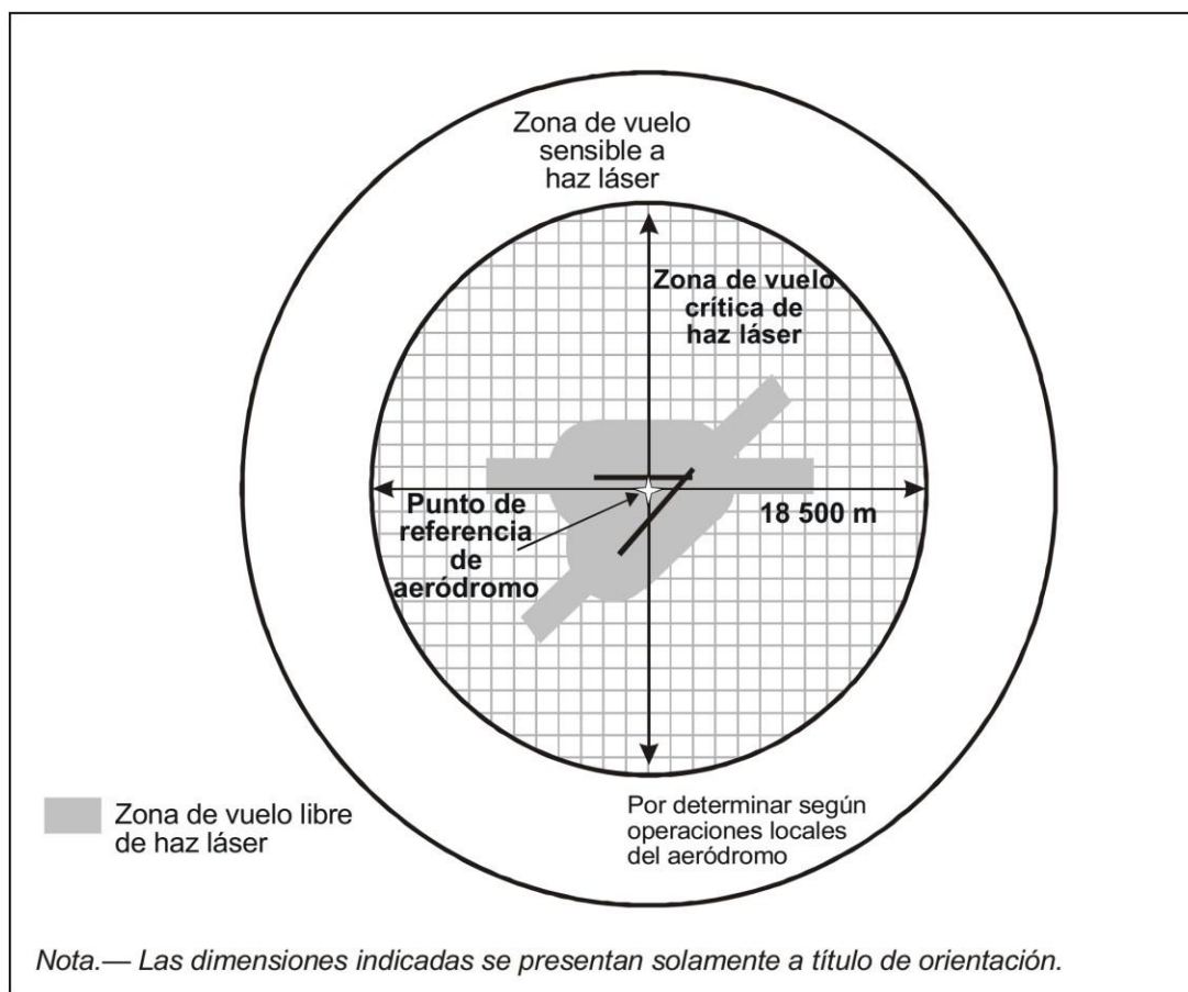
Figura D-1-1. Zonas de vuelo protegidas
