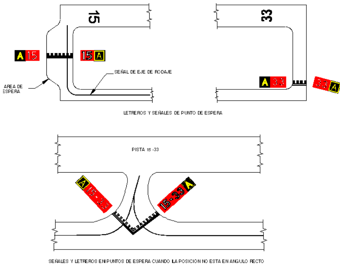
Figura 5. Letreos de posición de espera.
