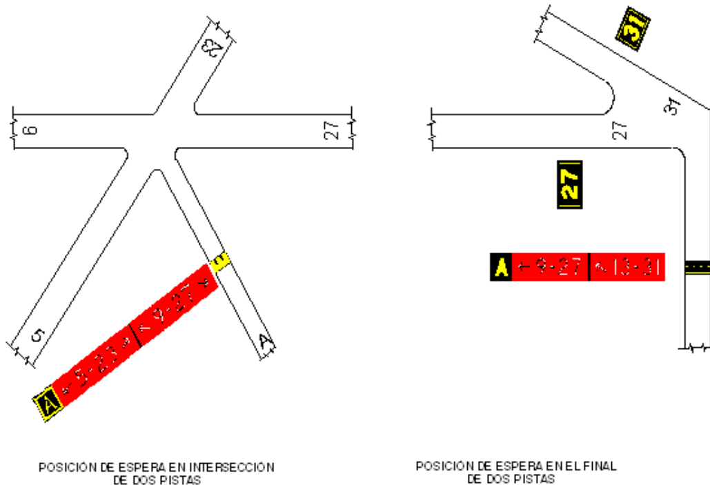
Figura 4. Letreros en puntos de espera de ingreso a pista
